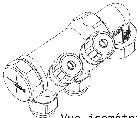
Vue isométrique Echelle : 1:2
